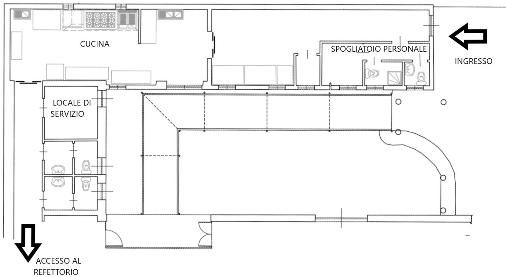
PLANIMETRIA CUCINA
